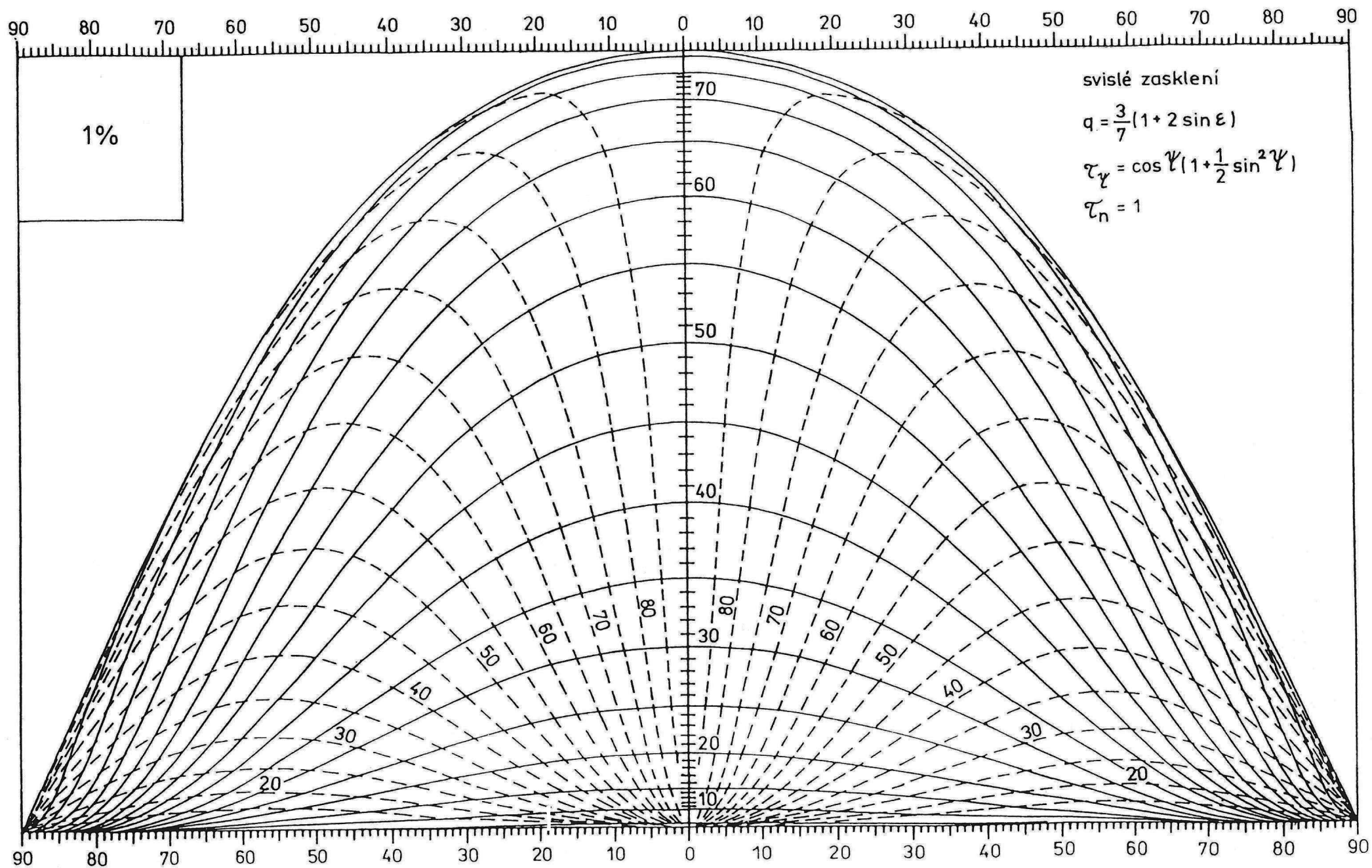
Waldramův diagram upravený pro osvětlení vodorovné roviny v interiéru
